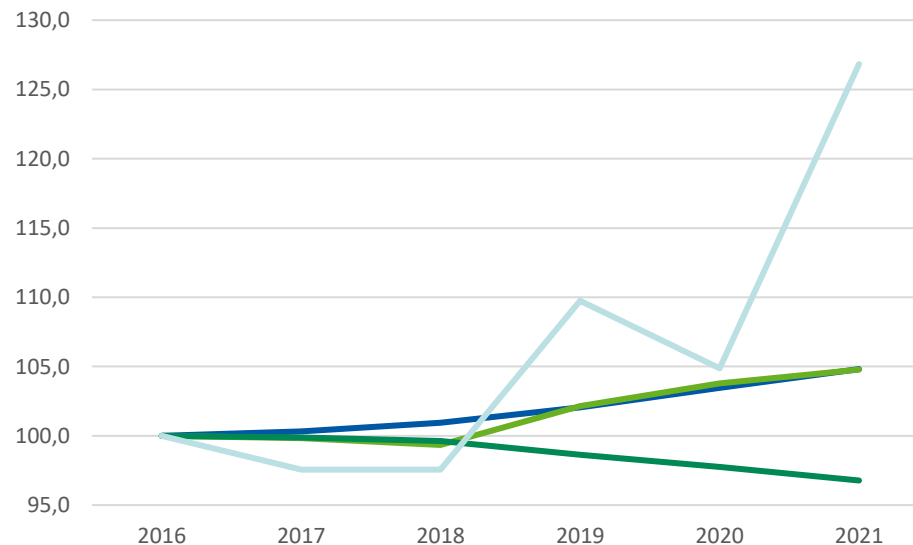
Relative Entwicklung von Siedlungsfläche, Verkehrsfläche, Vegetation und Gewässer in Bergisch Gladbach, 2016 = 100 %
