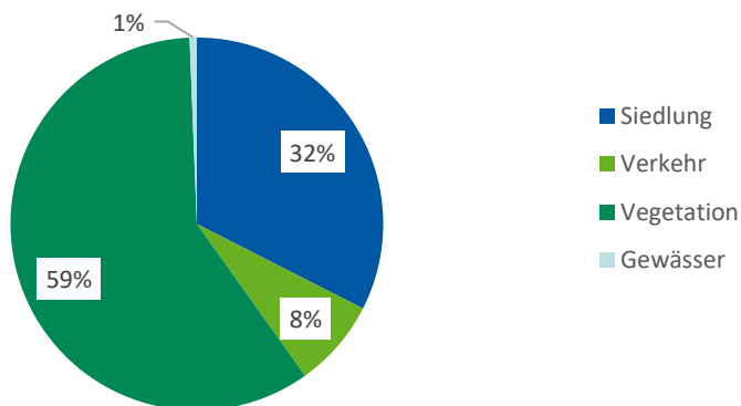
Anteile der Flächennutzungen an der Gesamtfläche in Bergisch Gladbach zum 31.12.2021
