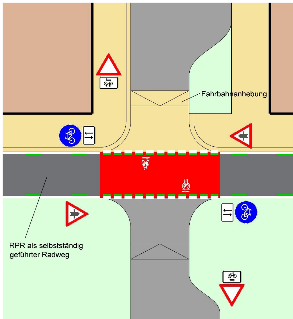
Abbildung 4-2: Bevorrechtigung im Zuge eines selbstständig geführten Weges
