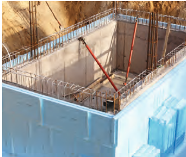
Keller in WU-Bauweise mit Wärmedämmschicht
