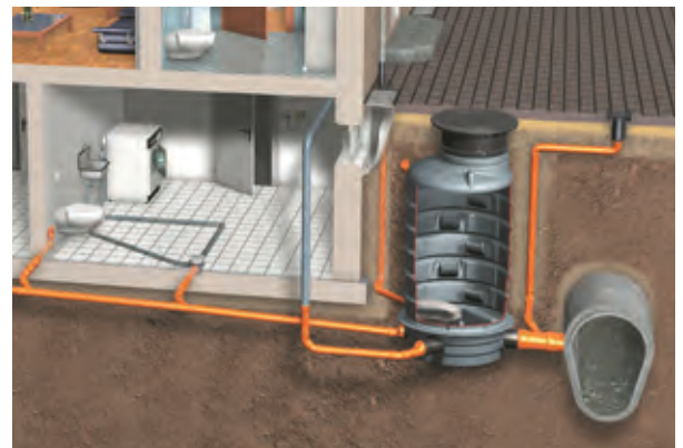
Rückstausicherung außerhalb des Gebäudes
