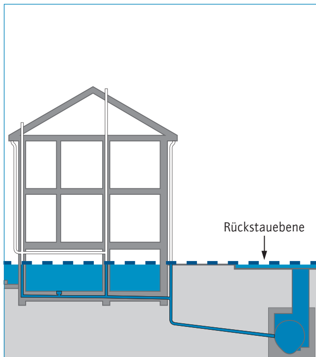
36 Rückstauenebene
